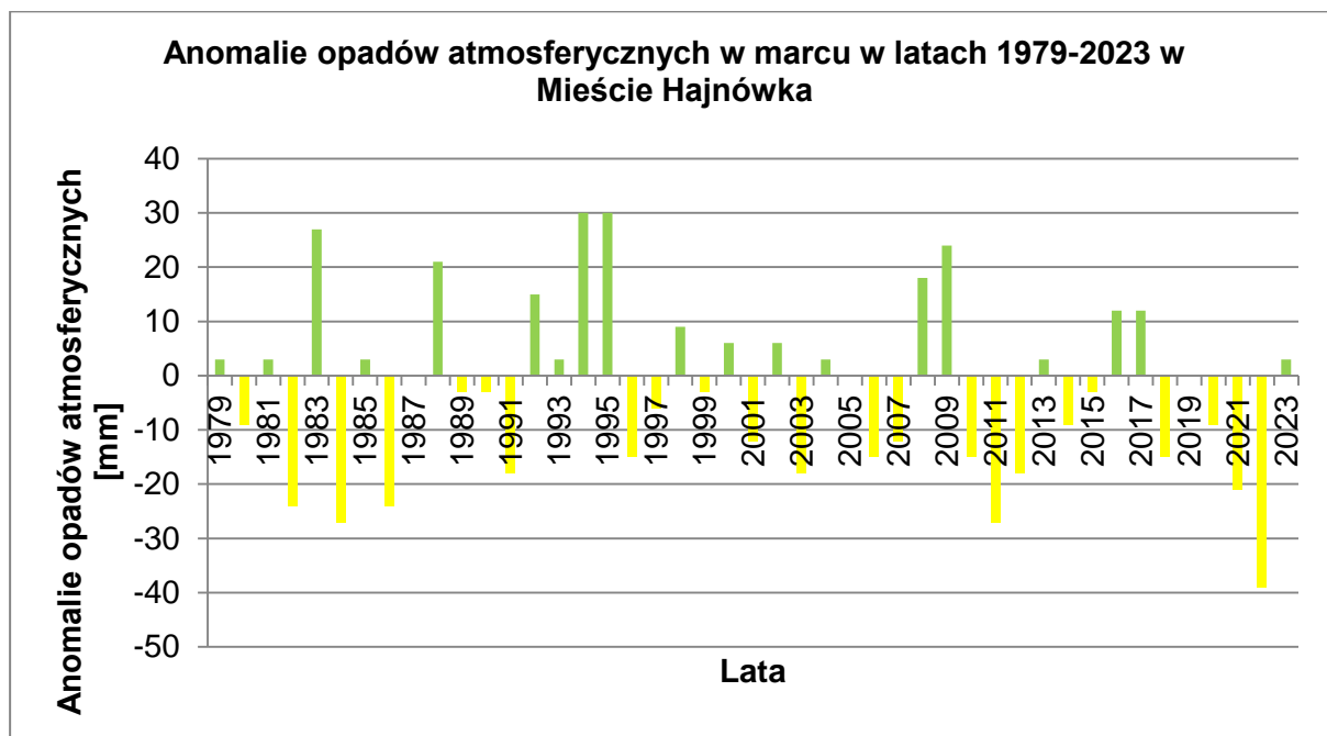
WYKRES 10 ANOMALIE OPADÓW ATMOSFERYCZNYCH W MARCU W LATACH 1979-2023 W MIEŚCIE HAJNÓWKA
