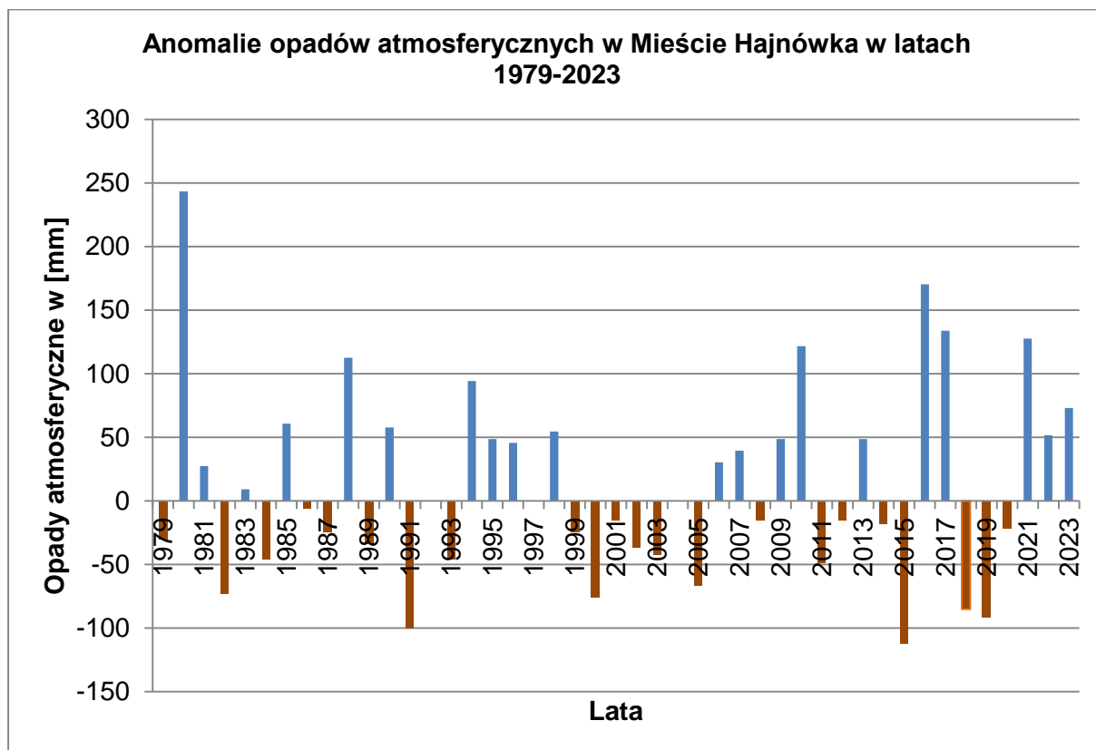
WYKRES 4 ANOMALIE OPADÓW ATMOSFERYCZNYCH W LATACH 1979-2023 W MIEŚCIE HAJNÓWKA
