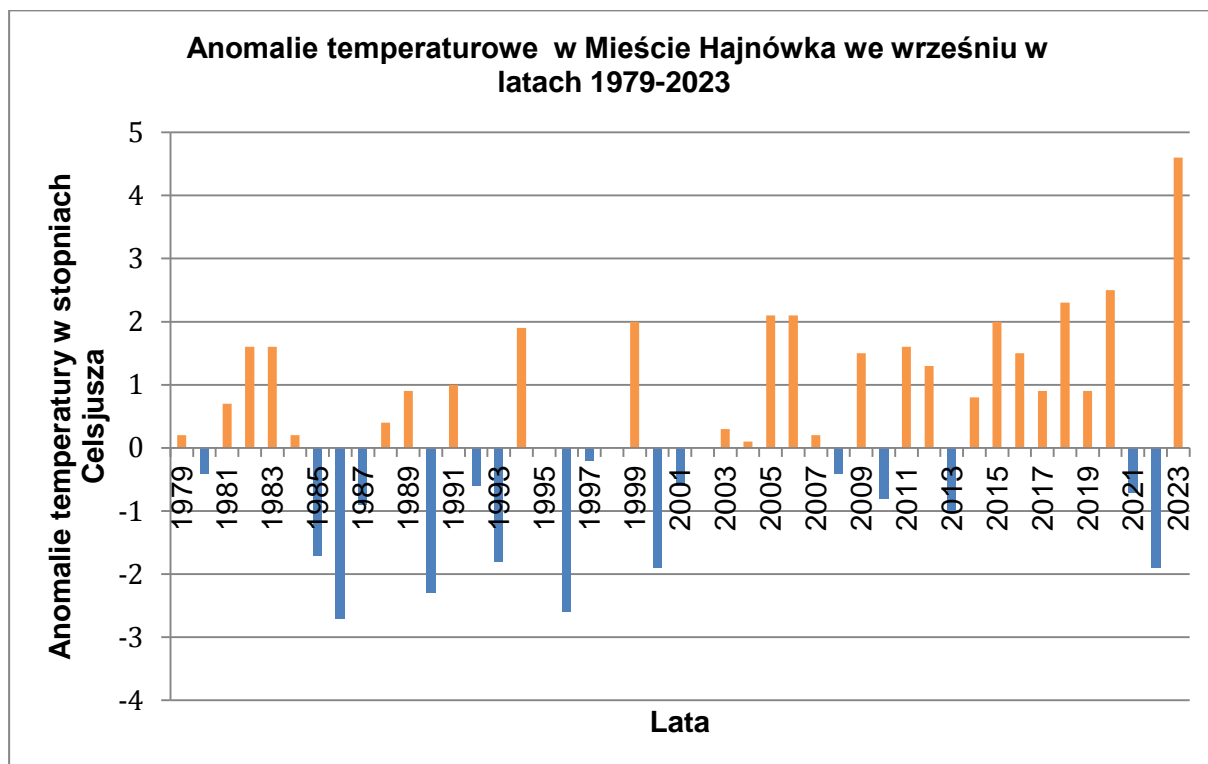
WYKRES 21 ANOMALIE TEMPERATUROWE WE WRZEŚNIU W LATACH 1979-2023 W MIEŚCIE HAJNÓWKA
