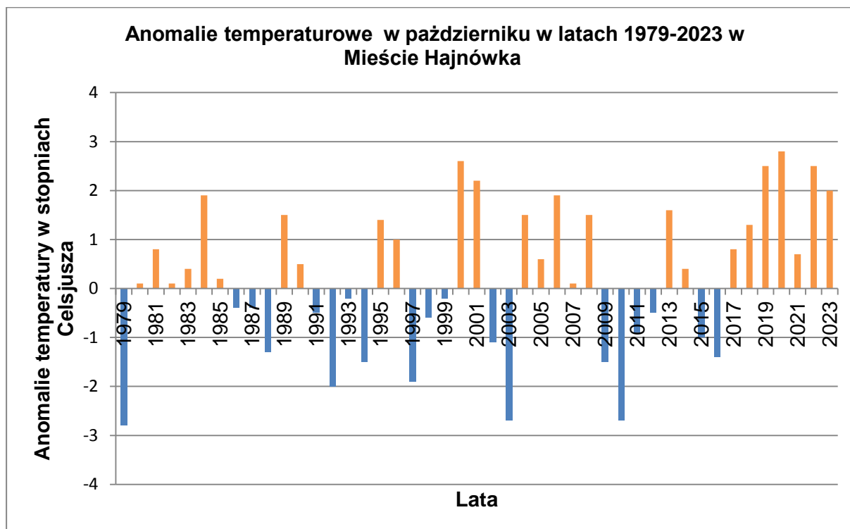
WYKRES 23 ANOMALIE TEMPERATUROWE W PAŹDZIERNIKU W LATACH 1979-2023 W MIEŚCIE HAJNÓWKA
