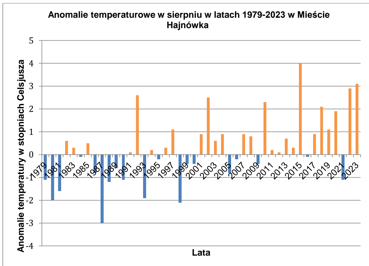
WYKRES 19 ANOMALIE TEMPERATUROWE W SIERPNIU W LATACH 1979-2023 W MIEŚCIE HAJNÓWKA
