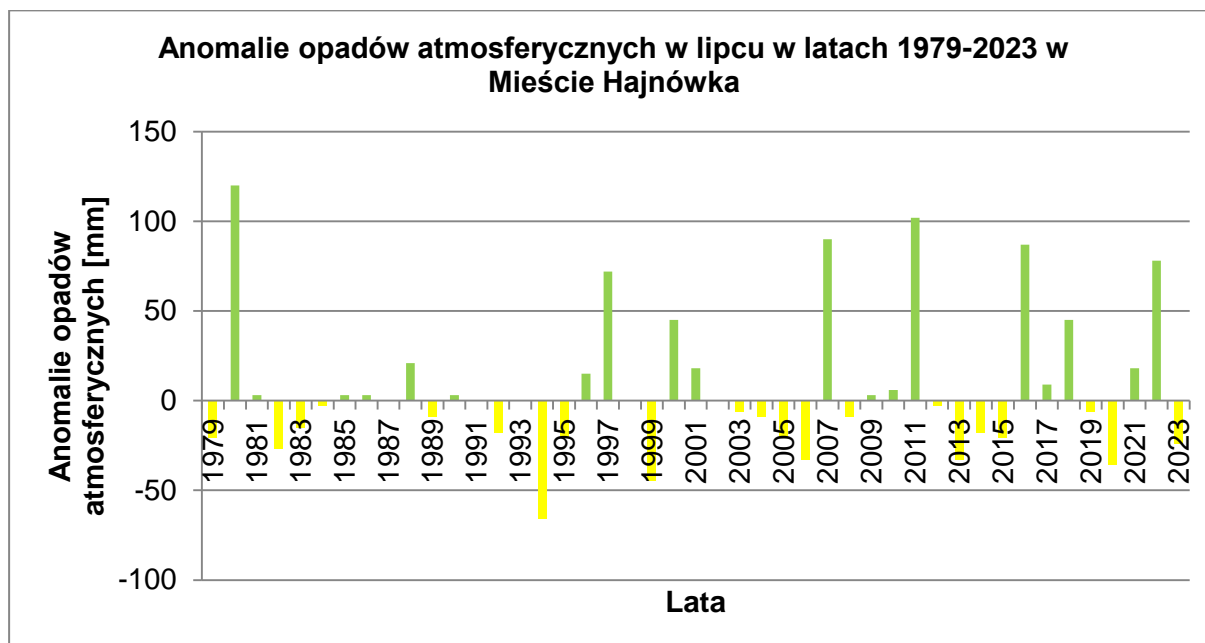
WYKRES 18 ANOMALIE OPADÓW ATMOSFERYCZNYCH W LIPCU W LATACH 1979-2023 W MIEŚCIE HAJNÓWKA
