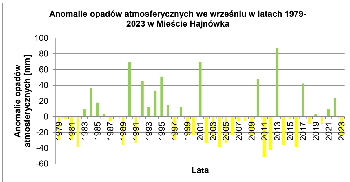
WYKRES 22 ANOMALIE OPADÓW ATMOSFERYCZNYCH WE WRZEŚNIU W LATACH 1979-2023 W MIEŚCIE HAJNÓWKA
