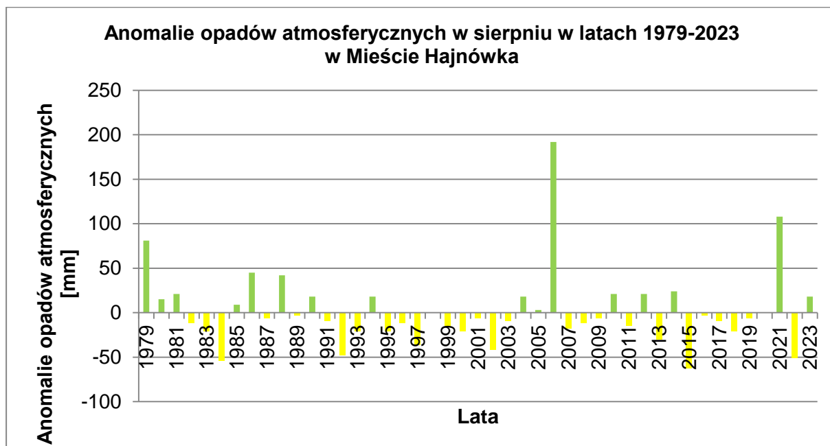
WYKRES 20 ANOMALIE OPADÓW ATMOSFERYCZNYCH W SIERPNIU W LATACH 1979-2023 W MIEŚCIE HAJNÓWKA
