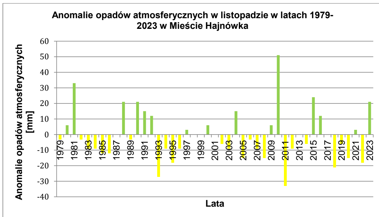
WYKRES 26 ANOMALIE OPADÓW ATMOSFERYCZNYCH W LISTOPADZIE W LATACH 1979-2023 W MIEŚCIE HAJNÓWKA
