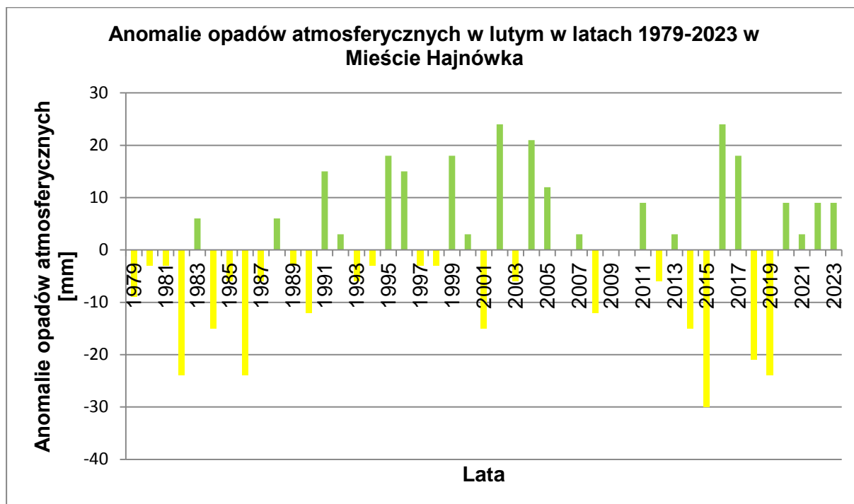
WYKRES 8 ANOMALIE OPADÓW ATMOSFERYCZNYCH W LUTYM W LATACH 1979-2023 W MIEŚCIE HAJNÓWKA
