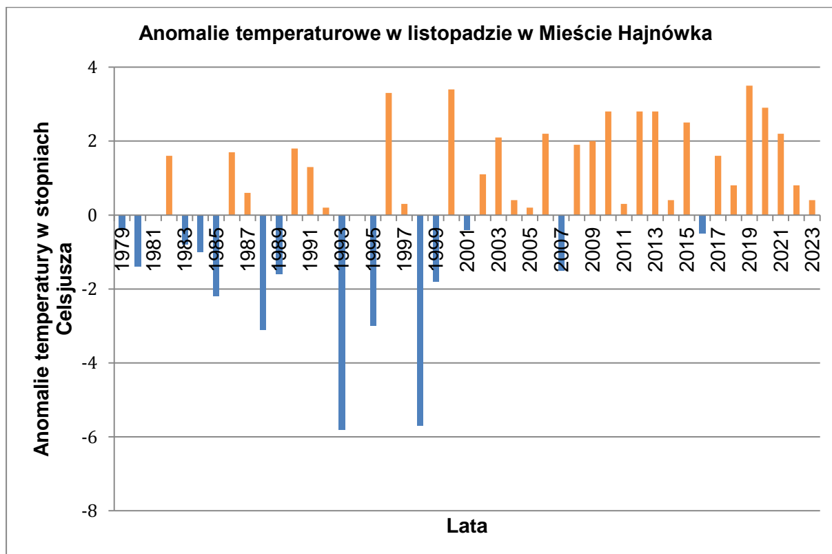
WYKRES 25 ANOMALIE TEMPERATUROWE W LISTOPADZIE W LATACH 1979-2023 W MIEŚCIE HAJNÓWKA
