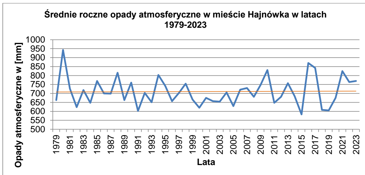
WYKRES 3 ŚREDNIE ROCZNE OPADY ATMOSFERYCZNE W MIEŚCIE HAJNÓWKA W LATACH 1979-2023
